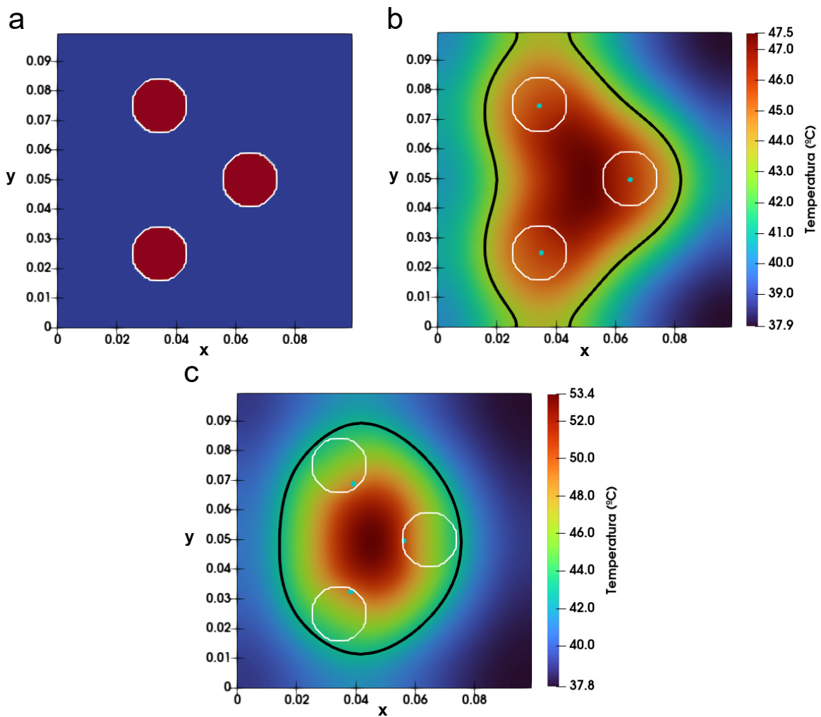
Figura 6.3: O tecido simulado e os resultados do terceiro cenário em duas dimensões. No Painel (a) a área vermelha representa o tecido tumoral, caso contrário, representa tecido saudável. O raio dos tumores é de 0,01m e os seus centros estão localizados respectivamente nos pontos (0,035; 0,025) , (0,065; 0,050) e (0,035; 0,075) . Os Painéis (b) e (c) apresentam a solução numérica da Equação (2.15) considerando uma exposição ao tratamento de hipertermia com t = 50min . No Painel (b) é apresentado o resultado que considera P_1 = (0,035; 0,025) , P_2 = (0,065; 0,050) e P_3 = (0,035; 0,075) , ou seja, os centros dos tumores. No Painel (c) é apresentado o resultado que considera os pontos que o processo de otimização encontrou, P_1 = (0,038338; 0,032350) , P_2 = (0,056189; 0,049626) e P_3 = (0,039135; 0,068854) . Os pontos azuis representam as posições P_1 , P_2 e P_3 , a linha preta sólida destaca a parte do domínio que atingiu T \geq 43^\circ , e o contorno branco sólido indica os limites do tumor.
