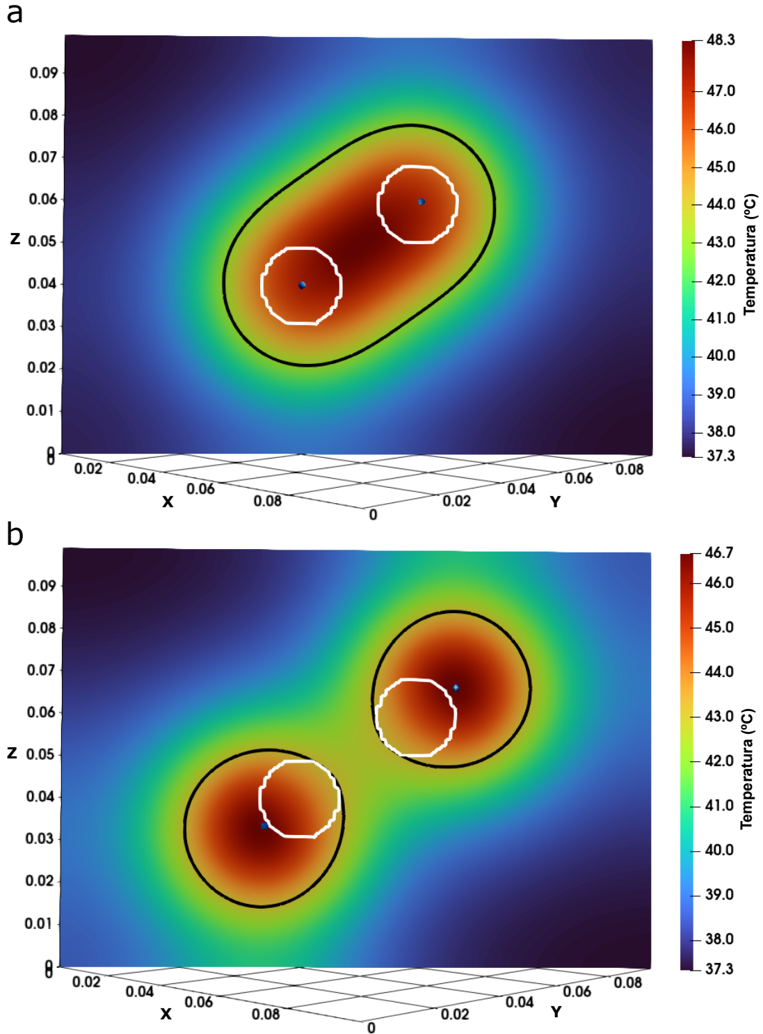
Figura 6.9: Corte no tecido considerando o plano x = -y . O contorno com a linha preta sólida destaca a porção do domínio que atingiu T \geq 43^\circ . O contorno em linha branca sólida indica a localização do tumor e os pontos azuis as posições das injeções. O painel (a) apresenta o resultado para a injeção posicionada no centro do tumor ( P_1 = (0,04; 0,04; 0,04) e P_2 = (0,06; 0,06; 0,06) ). O painel (b) apresenta o resultado para as injeções localizadas nos pontos obtidos pelo processo de otimização ( P_1 = (0,033357; 0,034644; 0,033353) e P_2 = (0,066553; 0,065626; 0,066493) ).
