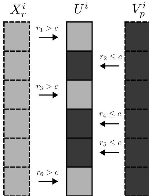
Figura 4.3: Representação do processo de crossover descrito na Equação (4.3), onde X_r^i , U^i e V_p^i são o vetor alvo, o vetor teste e o vetor de mutação, respectivamente.
